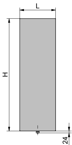
VZAPE Vooraanzicht
