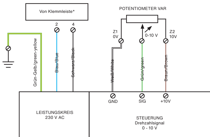
VAR - Abluftventilator (Fortluft)
