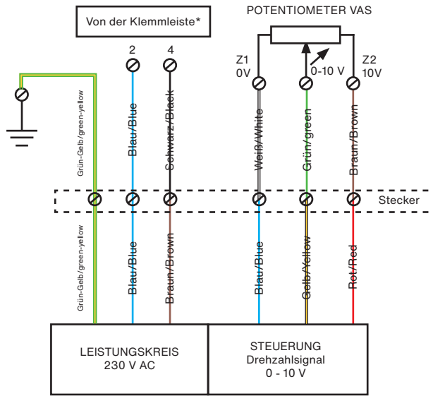
VAS - Zuluftventilator
