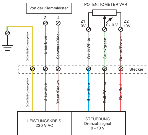
VAR - Abluftventilator (Fortluft)
