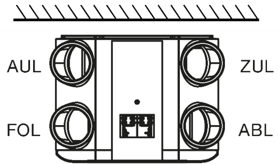
Zuluft und Abluft rechts
