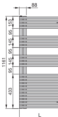
Pohled zepředu, LFAR-120
