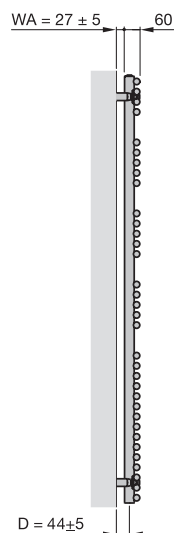
Pohled z boku, LFA(*)-170
