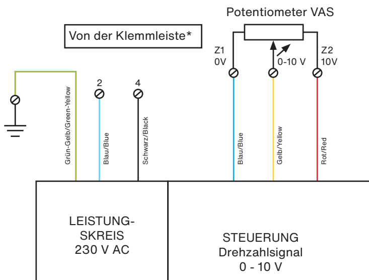
VAS - Zuluftventilator
