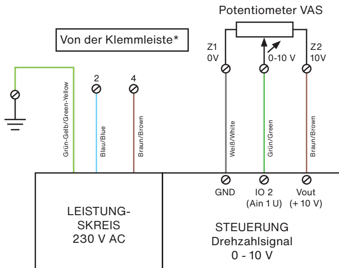
VAS - Zuluftventilator
