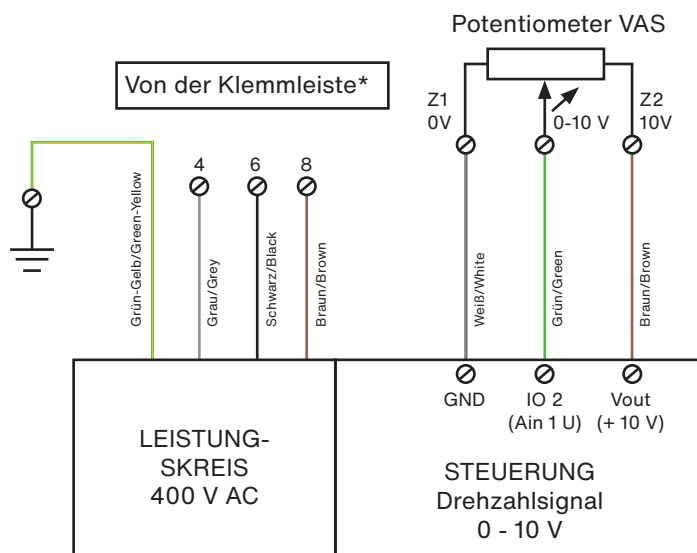
VAS - Zuluftventilator
