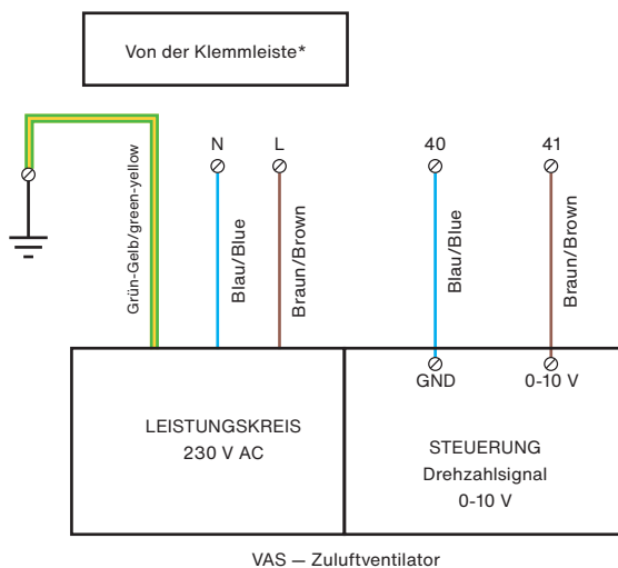
VAS – Zuluftventilator
