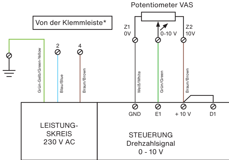
VAS - Zuluftventilator
