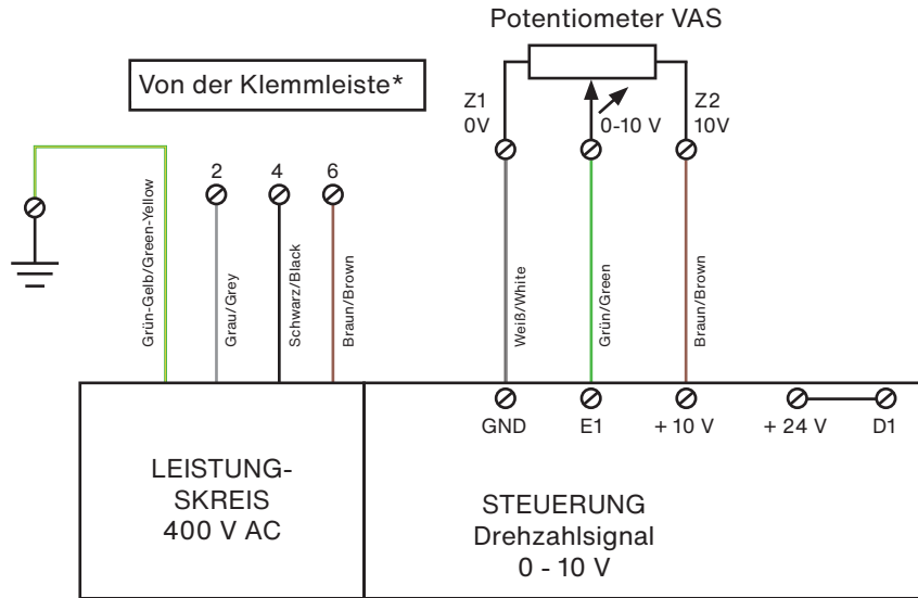
VAS - Zuluftventilator
