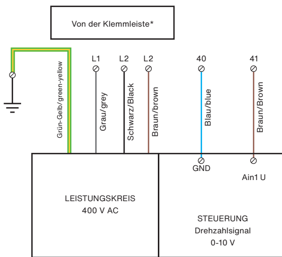
VAS – Zuluftventilator
