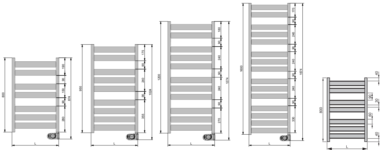
Pohled zepředu PQ6(C)-080
