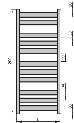
Pohled zepředu PQ6(C)-120
