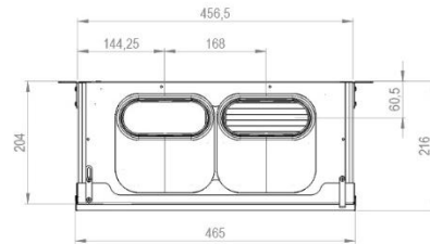
Wandaufputz- und Deckenmontage: Zu- und Abluftanschlüsse hinten
