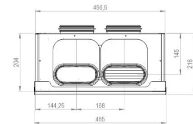
Wandaufputz- und wandintegrierte Montage: Zu- und Abluftanschlüsse vorne
