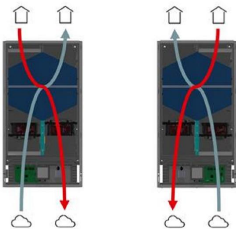
Rechtes Gerät (Zuluftanschluss rechts)
