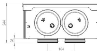
Wandaufputz- und wandintegrierte Montage: Außen- und Fortluftanschlüsse hinten
