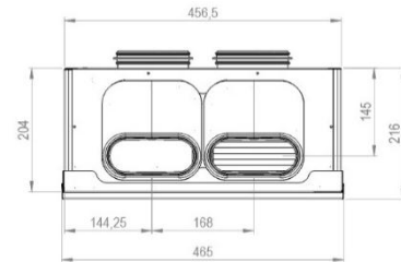
Wandaufputz- und wandintegrierte Montage: Zu- und Abluftanschlüsse vorne
