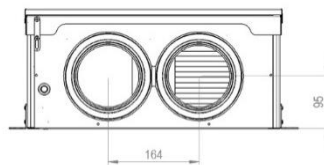
Wandaufputz- und Deckenmontage: Außen- und Fortluftanschlüsse unten
