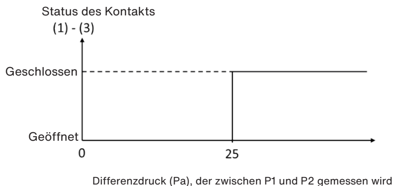
Zuluft-Druckschalter DEP S – Abluft-Druckschalter DEP R ECO - DIVA
