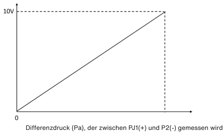
Druckgeber TRPS/TRPR LOBBY
