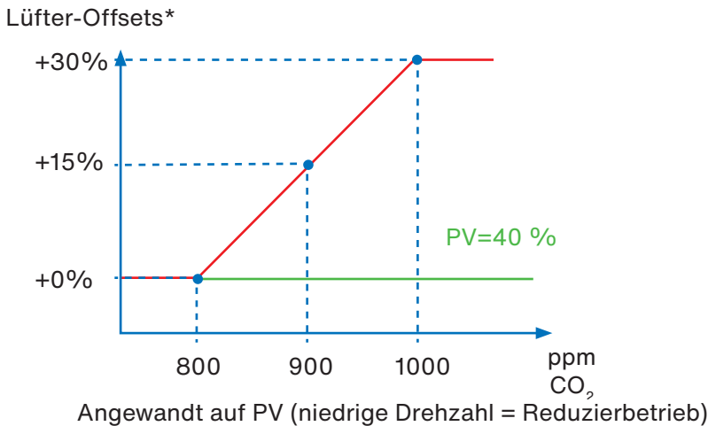
3 Offsets auf PV (niedrige Drehzahl) und lineare Interpolation
